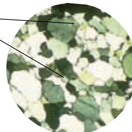
▲ Figura 8.15 La cuarcita es una roca metamórfica no foliada formada a partir de la arenisca rica en cuarzo. La microfotografía muestra los granos de cuarzo entrelazados típicos de la cuarcita. (Foto de E. J. Tarbuck.)
