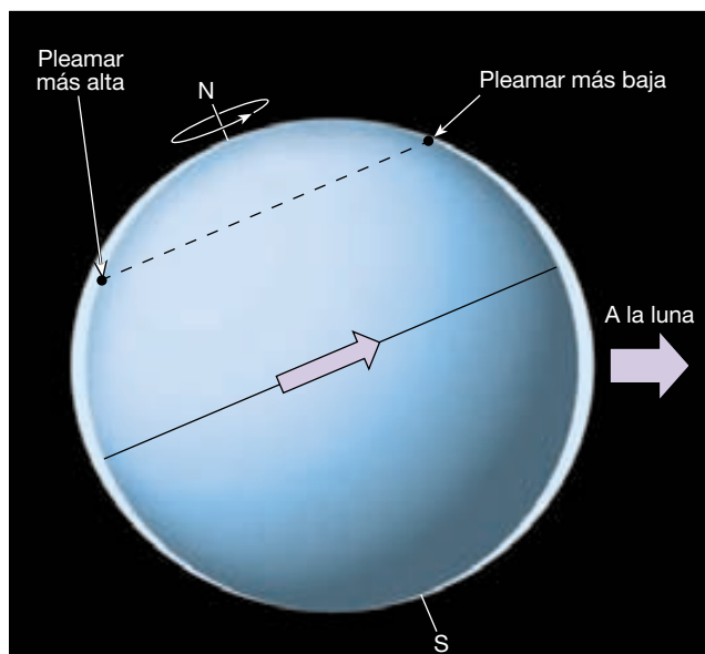
▲ Figura 20.16 Pandeos mareales idealizados en la Tierra provocados por la Luna. Si la Tierra estuviera cubierta a una profundidad uniforme por agua, habría dos pandeos mareales: uno en el lado de la Tierra orientado a la Luna (derecha) y otro en el lado opuesto de la Tierra (izquierda). Dependiendo de la posición de la Luna, los pandeos mareales pueden inclinarse hacia el ecuador de la Tierra. En esta situación, la rotación de la Tierra hace que un observador experimente dos mareas altas desiguales durante un día.
