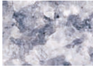
▲ Figura 7.8 Como otras evaporitas, esta muestra de salgema se dice que tiene una textura no clásica porque está compuesta de un intercrecimiento de cristales.
