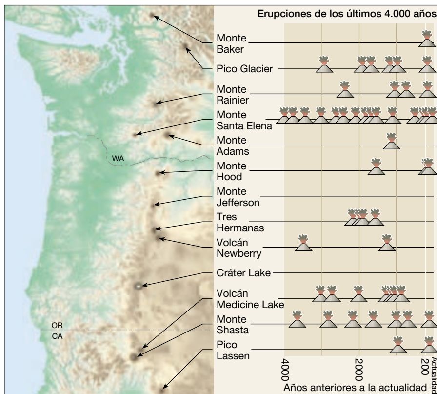
Figura 5.9 De los 13 volcanes potencialmente activos de la cordillera Cascade, 11 han hecho erupción en los últimos 4.000 años y 7 en sólo los últimos 200 años. Más de 100 erupciones, la mayoría de las cuales fueron explosivas, han sucedido en los últimos 4.000 años. El Santa Elena es el volcán más activo de la cordillera Cascade. Sus erupciones han oscilado entre expulsiones de lava relativamente tranquilas a acontecimientos explosivos mucho mayores que el del 18 de mayo de 1980. Cada símbolo de erupción en el diagrama representa de una a doce erupciones en muy poco espacio de tiempo. (Tomado de U. S. Geological Survey.)
